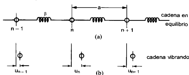
Figura 4. Esquema de una cadena lineal monoatómica unidimensional. (a) en equilibrio; (b) vibrando, con los átomos desplazados.
