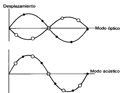
Figura 9. Los desplazamientos atómicos asociados a las vibraciones de una red biatómica: (a) de la rama óptica, (b) de la rama acústica. De nuevo, por claridad, se han representado los desplazamientos transversales en lugar de los longitudinales.
