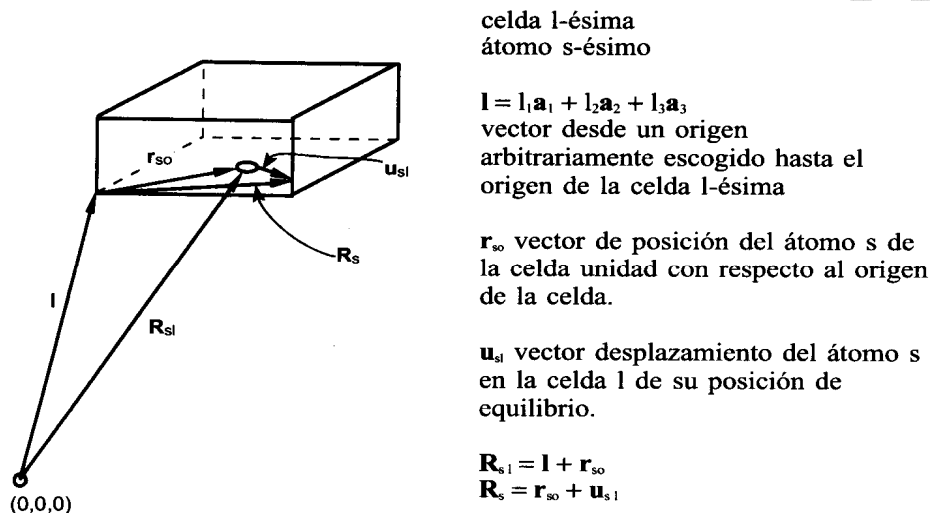
Figura 11. Ilustración de la notación utilizada.
