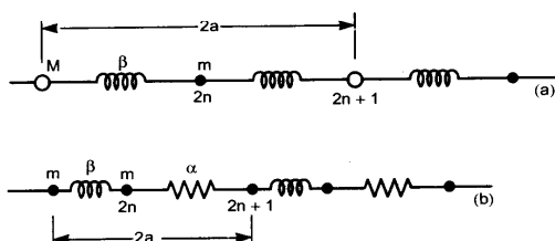
Figura 7. (a) Cadena unidimensional biatómica formada por átomos diferentes conectados por fuerzas recuperadoras idénticas. (b) Cadena lineal biatómica formada por átomos idénticos conectados por fuerzas recuperadoras diferentes.
