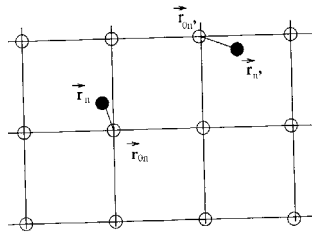
Figura 3. Notación de los átomos en equilibrio en los nudos de la red de Bravais y de los desplazamientos asociados.
