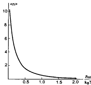
Figura 16. Número medio de fonones por modo, \langle n \rangle , en función de x = \hbar\omega/k_B T
